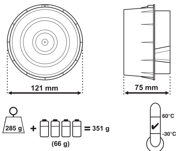
Figura 1: Montaggio B501RF
