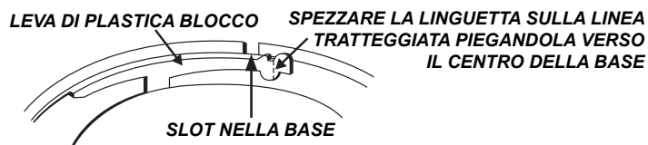
Figura 3b: Rimozione della sirena dalla base
