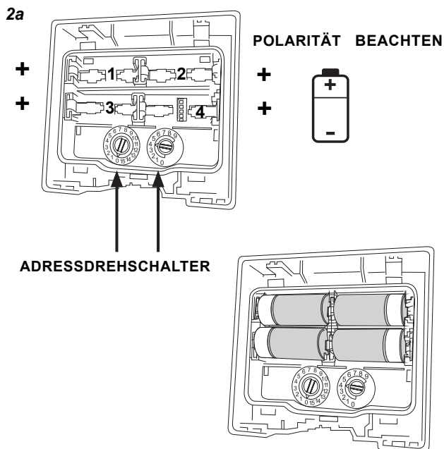
Abbildung 2: Installation der Batterien und Lage der Adressdrehesalter
