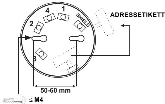
Abbildung 1: B501AP Montage
