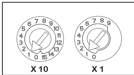
Abbildung 4: Adressdrehschalter
