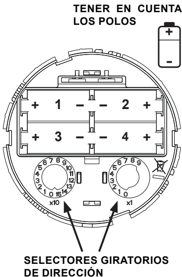
Figura 4: Instalación de las pilas y selectores giratorios de dirección
