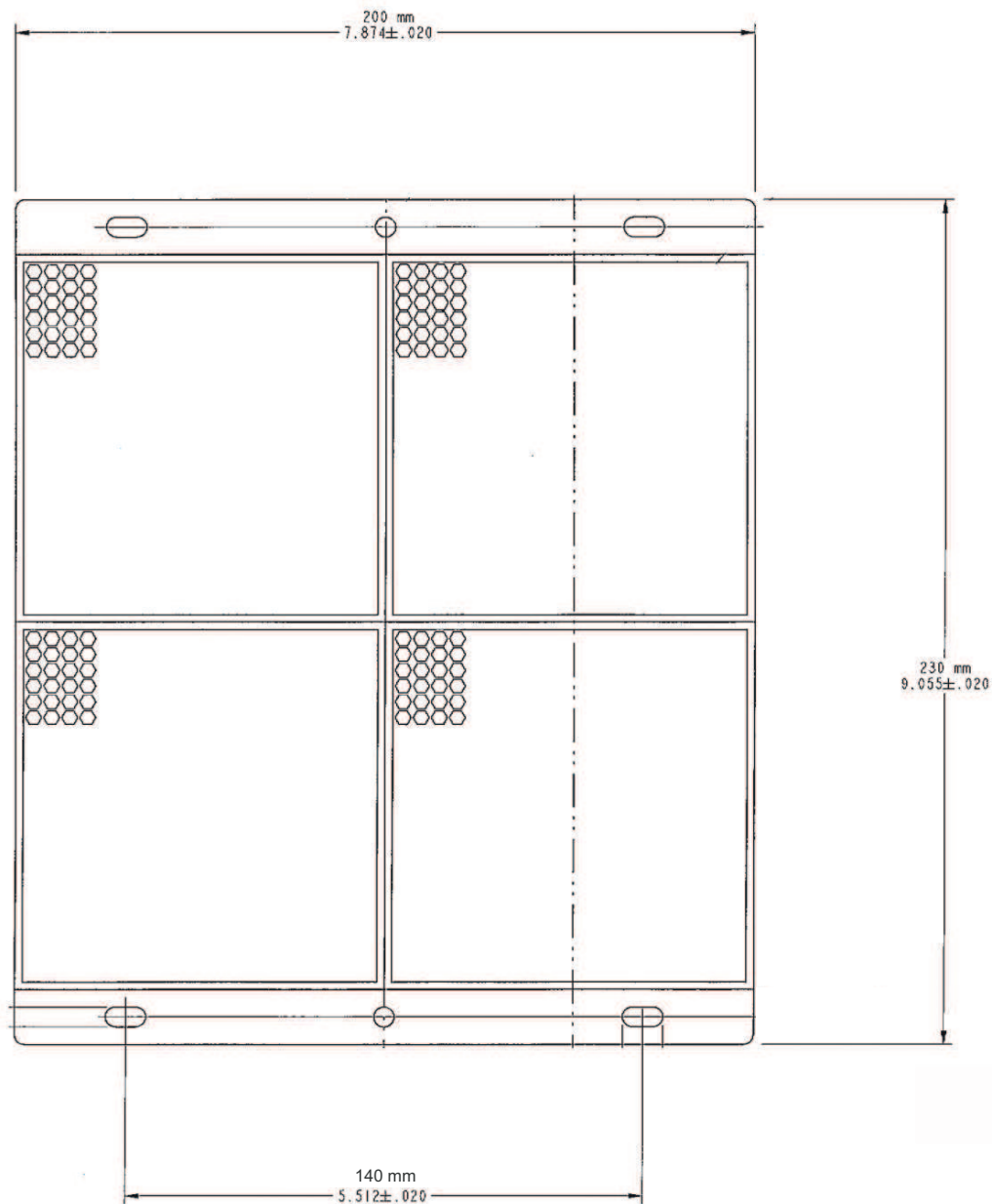
Afbeelding 3-2: Afmetingen reflector
