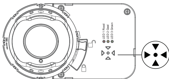
Afbeelding 3-19: Pijltjesopstelling
