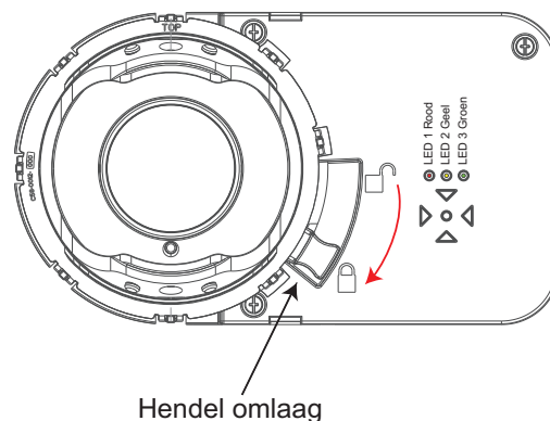
Afbeelding 3-21: De oogbol vergrendelen en beveiligen
