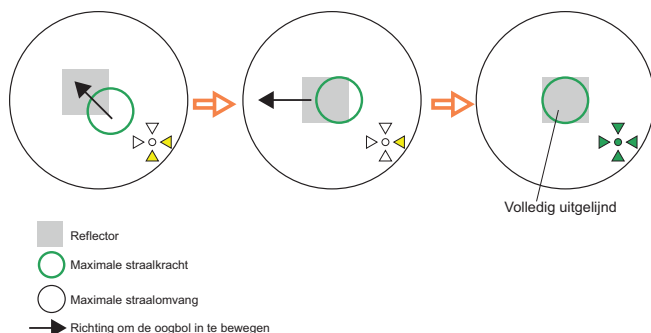
Afbeelding 3-20: Uitlijningshulpmiddel met gekleurde pijltjesopstelling
