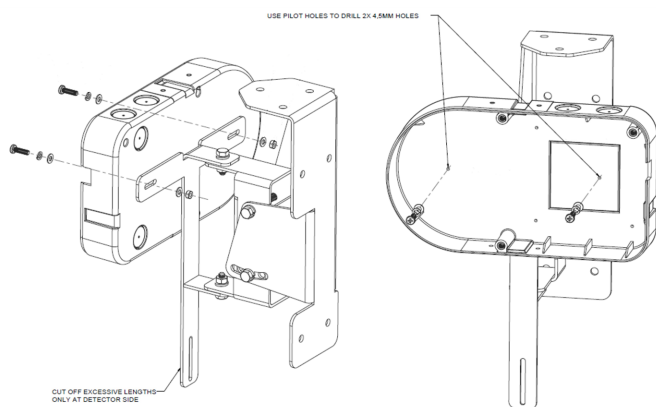
Afbeelding 3-12: Montagerichtlijnen detector
