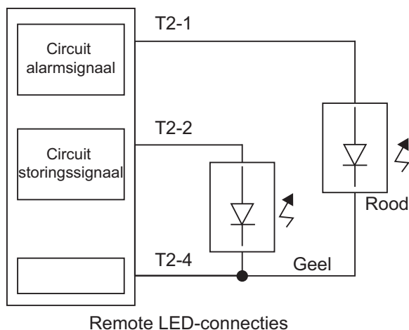
Afbeelding 3-16: Bekabelingsschema (remote LED's)
