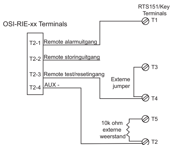
Afbeelding 3-14: Bekabelingsschema
