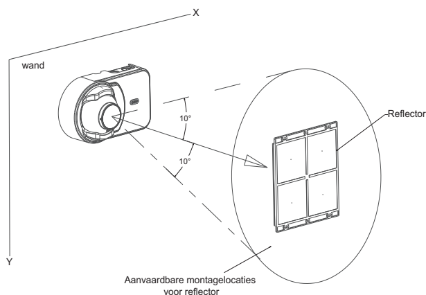
Afbeelding 3-8: Montagerichtlijnen reflector
