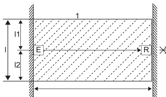
Afbeelding 3-7: Te bewaken ruimte
