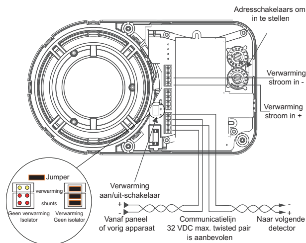
Afbeelding 3-14: Bekabelingsschema
