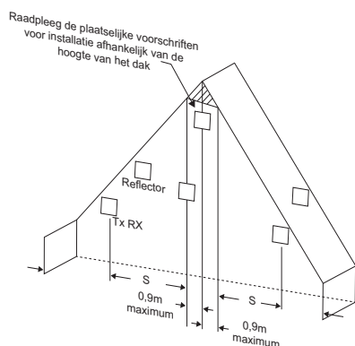
Afbeelding 3-6: Schuin plafond (type punt)
