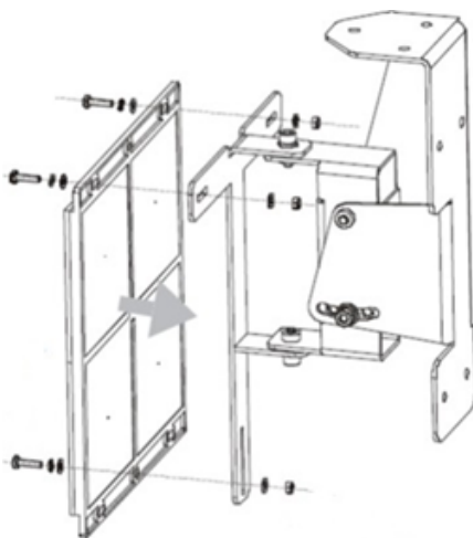
Afbeelding 3-9: Montagerichtlijnen reflector
