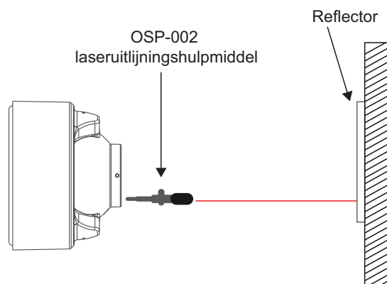
Afbeelding 3-17: Globale uitlijning
