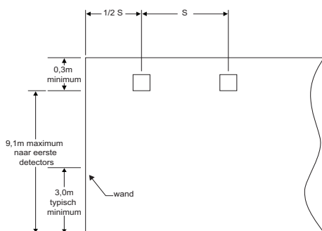
Afbeelding 3-3: Glad plafond (zij-aanzicht)
