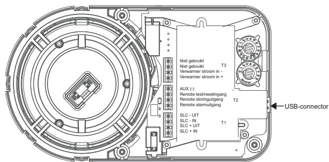
Afbeelding 3-13: Bekabelingsverbindingen bij detector
