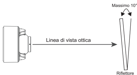
Figura 2-5: Linee guida per il montaggio del riflettore
