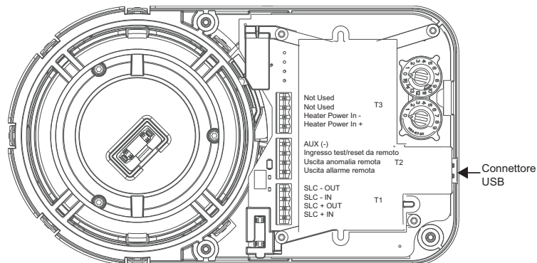
Figura 2-8: Connessioni elettriche presso il rivelatore
