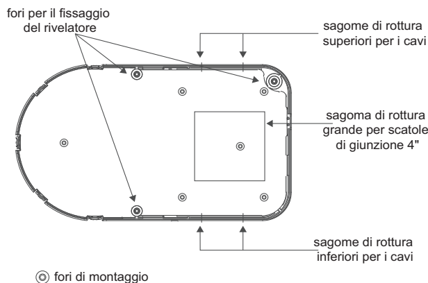
Figura 2-6: Fori di guida per il montaggio
