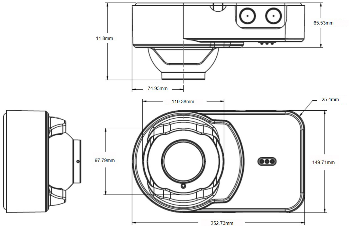
Figura 2-1: Dimensioni rivelatore
