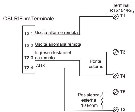
Figura 2-9: Schema elettrico
