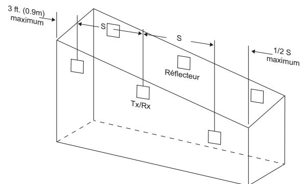
Figure 3-5: Plafond en pente (type dents de scie)
