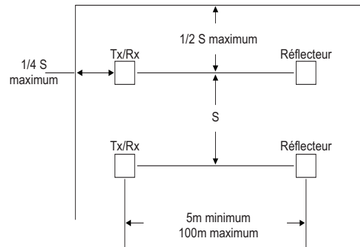
Figure 3-4: Plafond lisse (vue de dessus)
