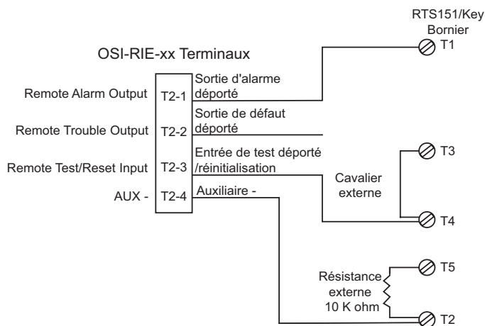
Figure 3-15: Schéma de câblage (RTS151)
