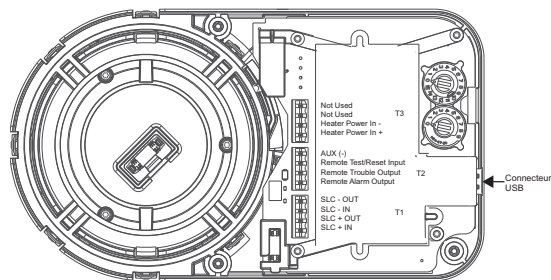
Figure 3-13: Raccords de câblage au détecteur
