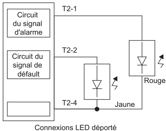
Figure 3-16: Schéma de câblage (voyants LED à distance)
