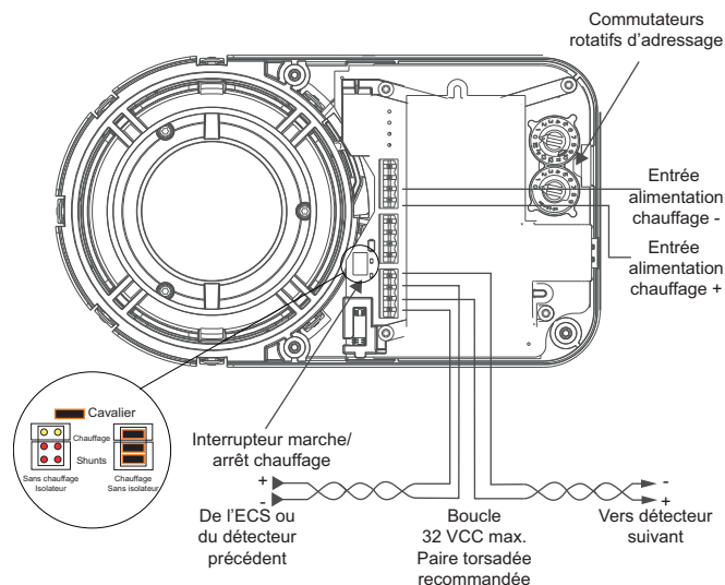
Figure 3-14: Schéma de câblage
