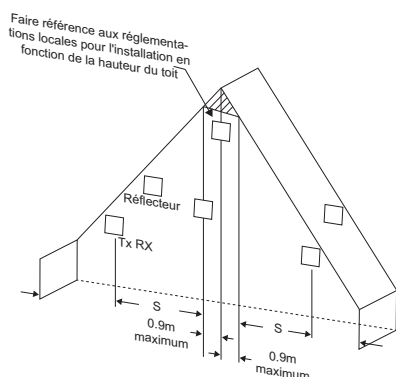
Figure 3-6: Plafond en pente (type en pointe)
