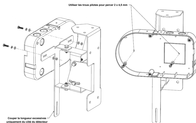
Figure 3-12: Directives de montage du détecteur
