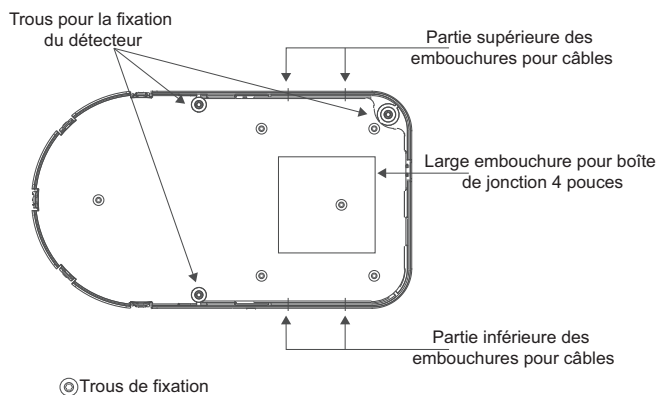
Figure 3-11: Montage des trous pilotes
