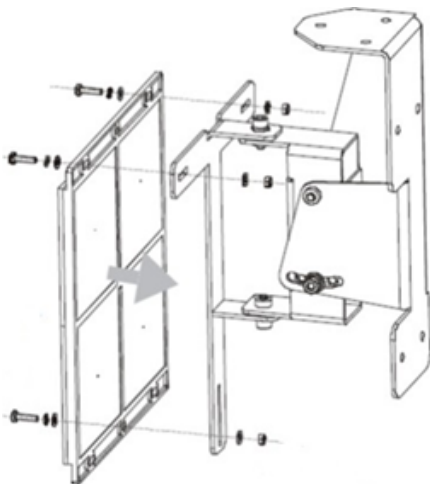
Figure 3-9: Directives de montage du réflecteur avec le kit multi-montage
