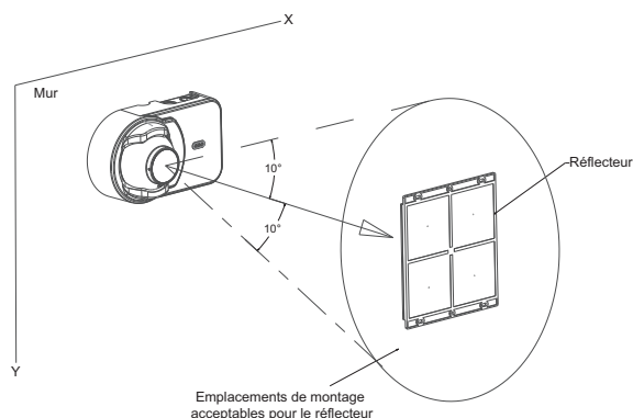
Figure 3-8: Directives de montage du réflecteur
