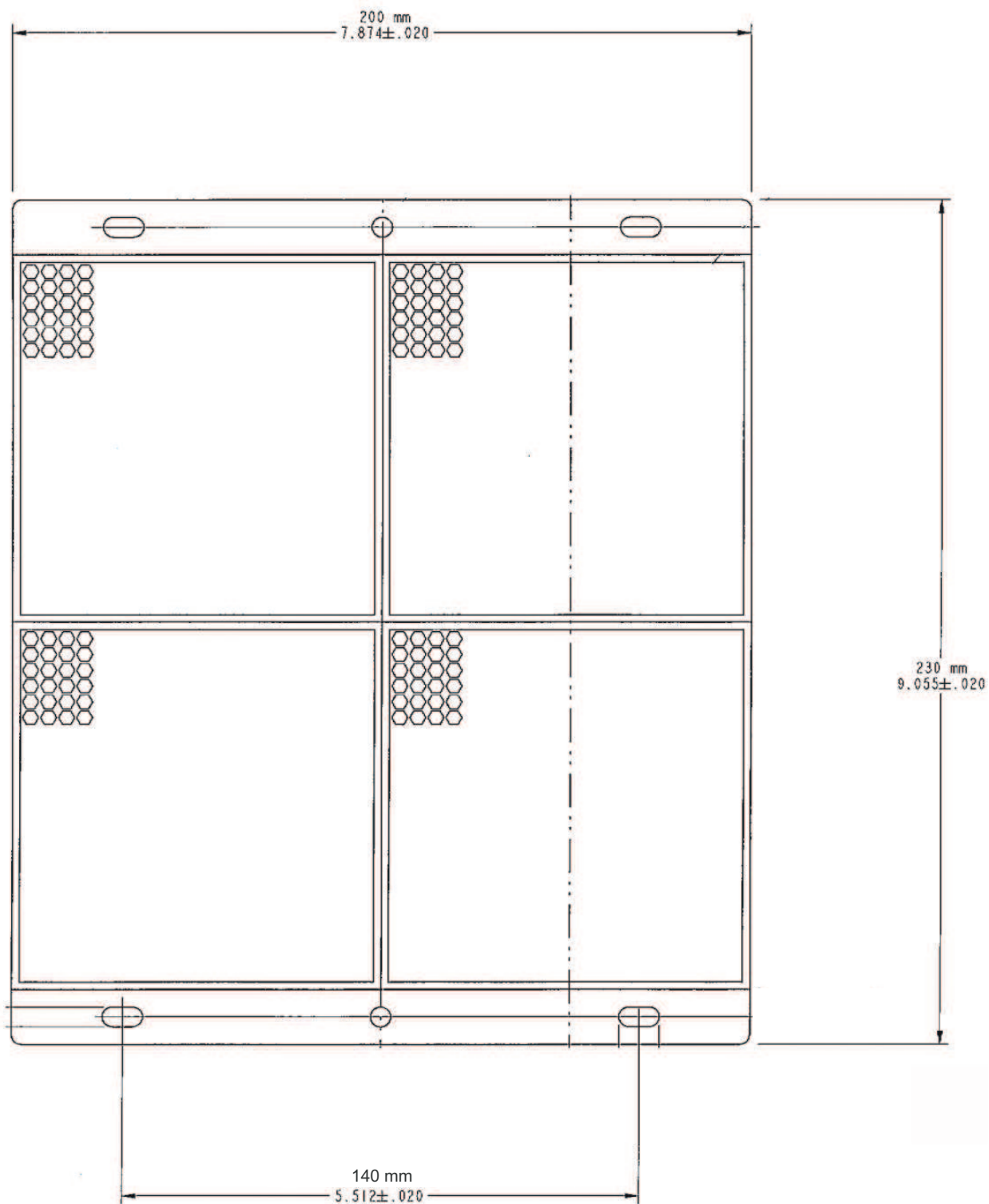
Figure 3-2: Dimensions du réflecteur
