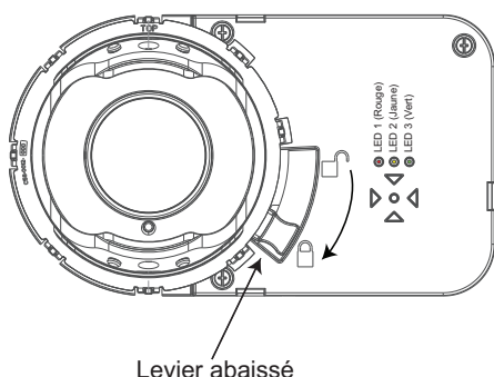
Figure 3-21: Verrouillage et fixation du globe
