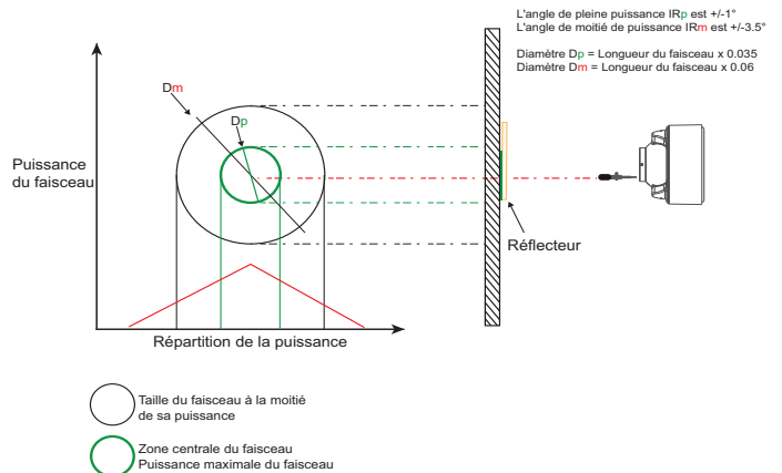
Figure 3-18: Répartition de la puissance du faisceau
