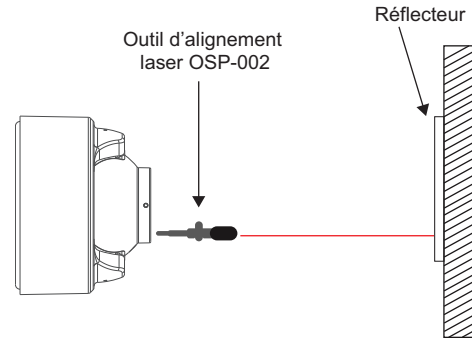
Figure 3-17: Alignement grossier
