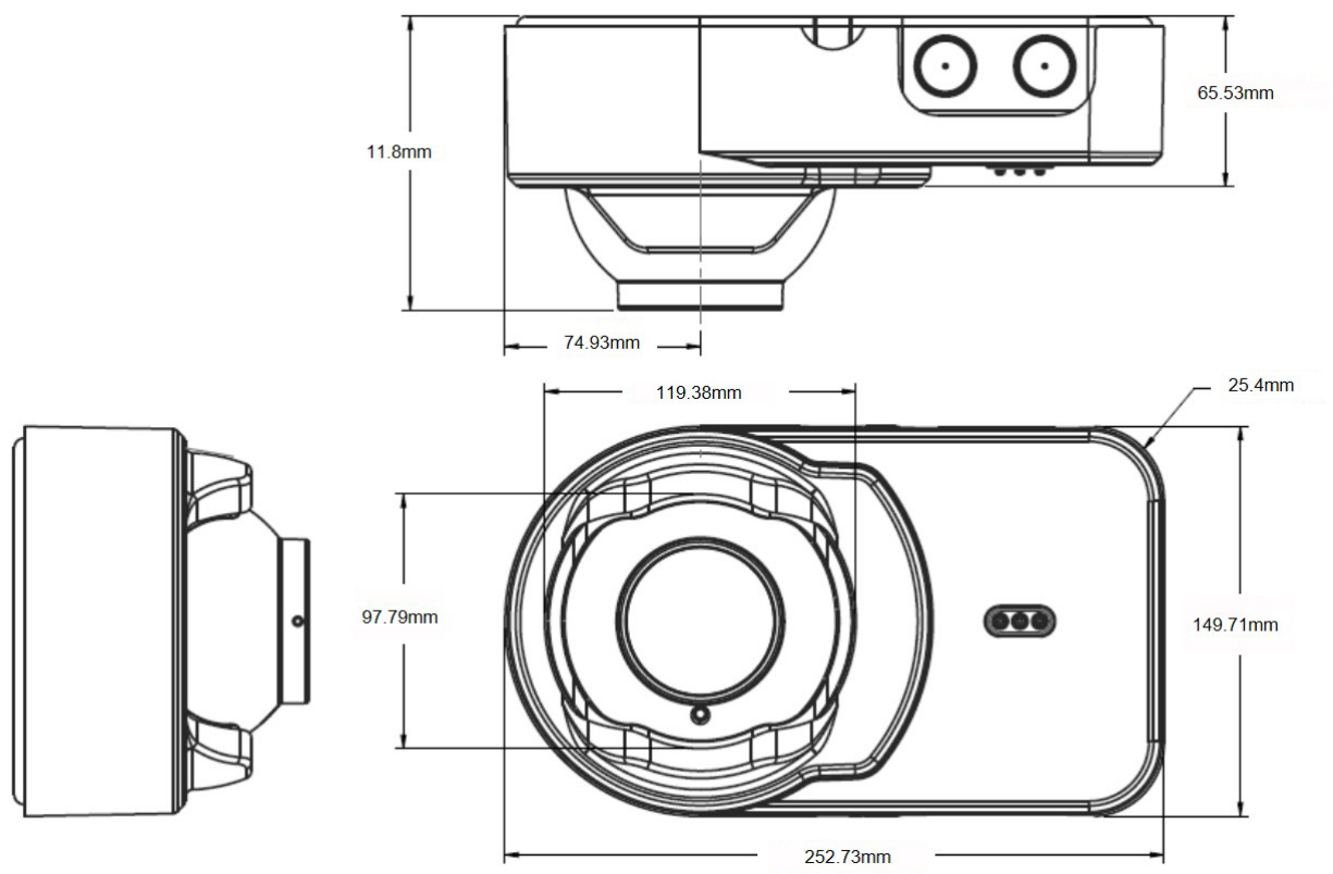
Figure 3-1: Dimensions du détecteur
