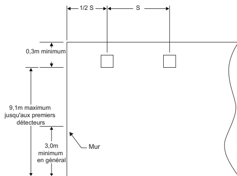
Figure 3-3: Plafond lisse (vue latérale)
