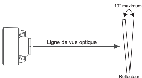
Figure 3-10: Directives de montage du réflecteur
