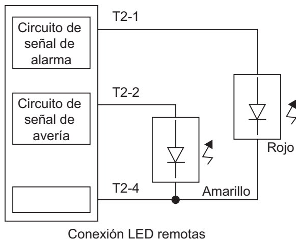
Figura 3-14: Diagrama de cableado (LED remotos)
