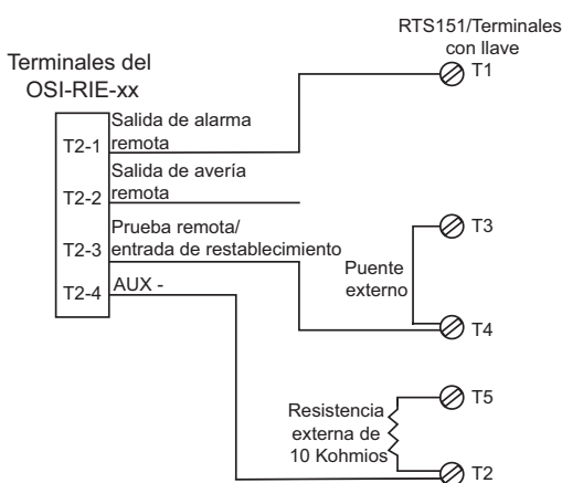
Figura 3-12: Diagrama de cableado
