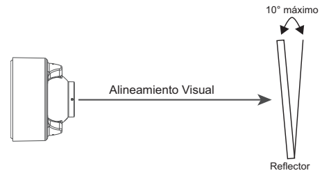
Figura 3-8: Instrucciones de montaje del reflector
