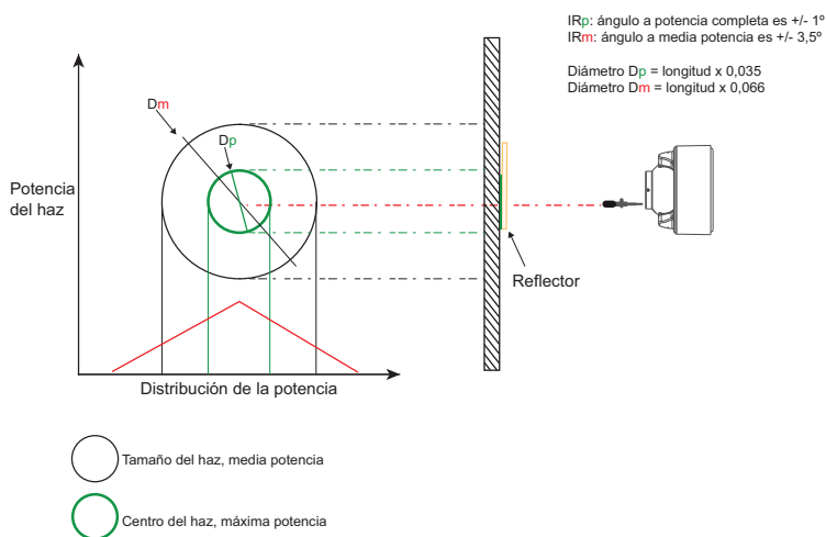
Figura 3-16: Distribución de potencia del haz
