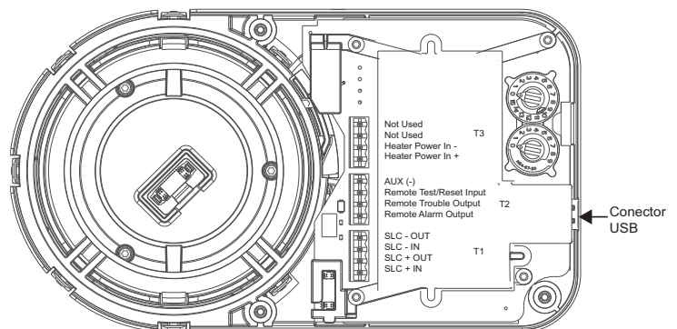
Figura 3-11: Conexiones de cableado en el detector
