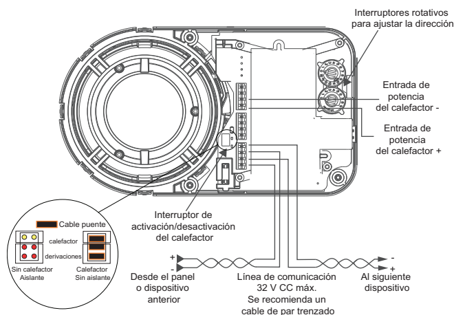
Figura 3-12: Diagrama de cableado
