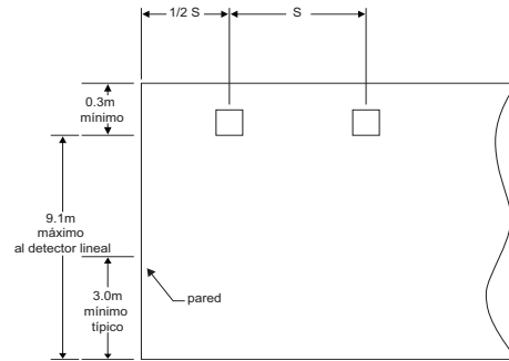
Figura 3-1: Techo liso (vista lateral)
