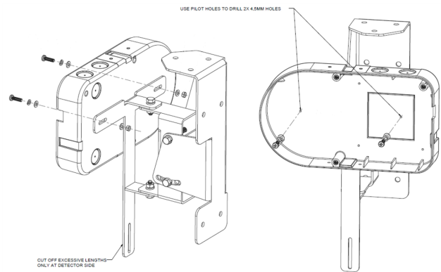
Figura 3-10: Instrucciones de montaje del detector
