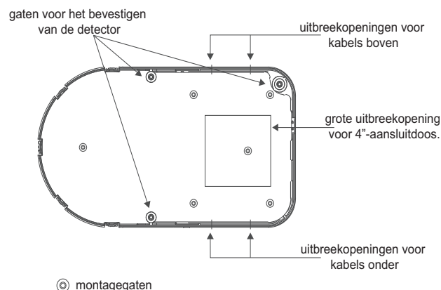
Afbeelding 2-11: Geleidegaten voor montage
