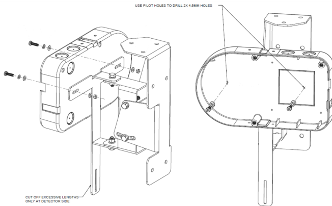
Afbeelding 2-12: Montagerichtlijnen detector
