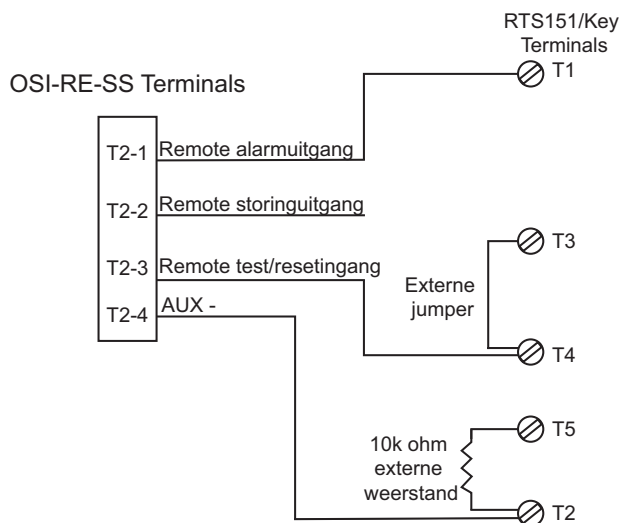
Afbeelding 2-15: Bekabelingsschema (RTS451 of RTS151)
