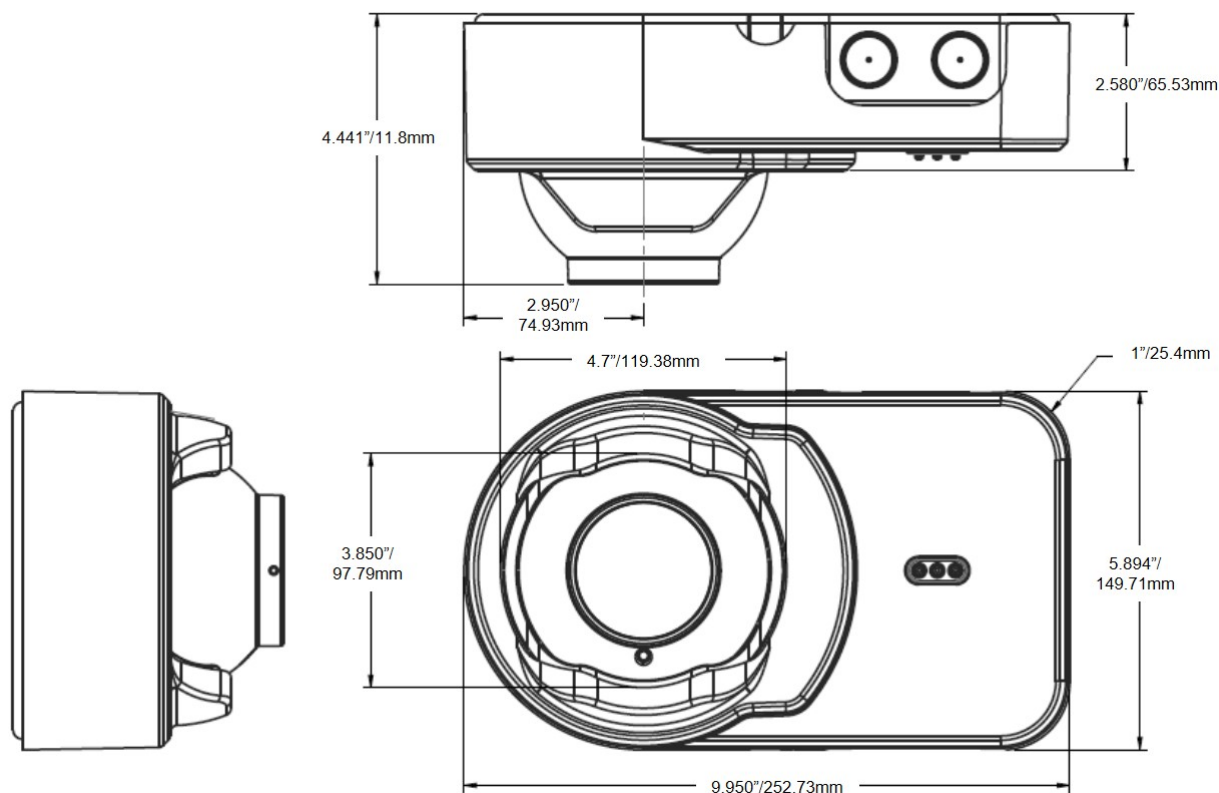
Afbeelding 2-1: Afmetingen detector
