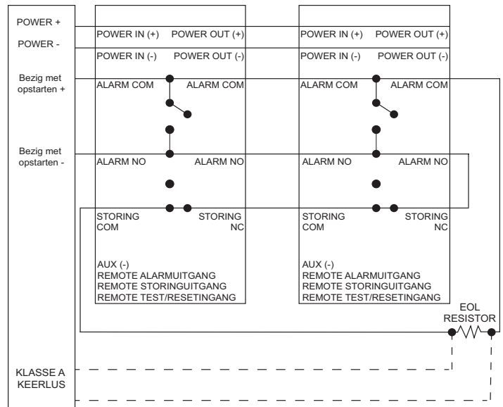
Afbeelding 2-13: Bedradingsschema
