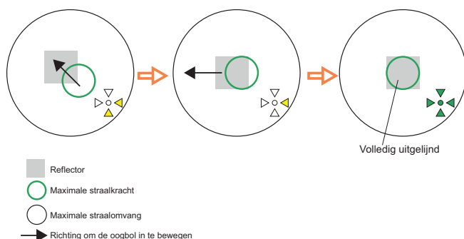
Afbeelding 2-20: Uitlijningshulpmiddel met gekleurde pijltjesopstelling
