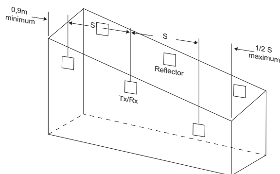
Afbeelding 2-5: Schuin plafond (type schuur)
