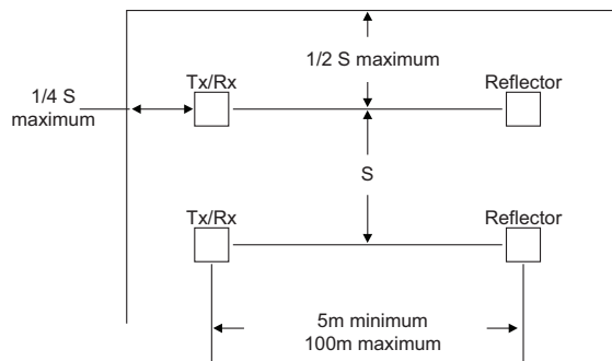
Afbeelding 2-4: Glad plafond (bovenaanzicht)
