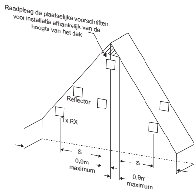
Afbeelding 2-6: Schuin plafond (type punt)
