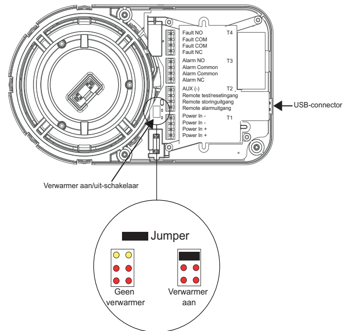
Afbeelding 2-14: Bedradingsverbindingen bij detector
