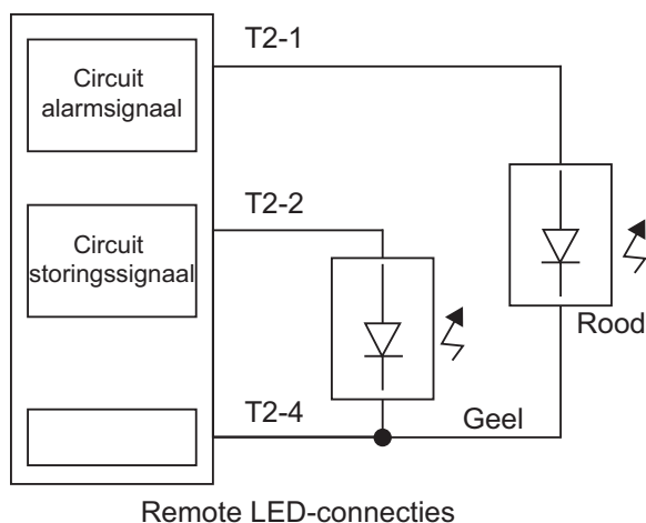
Afbeelding 2-16: Bekabelingsschema (remote LED's)
