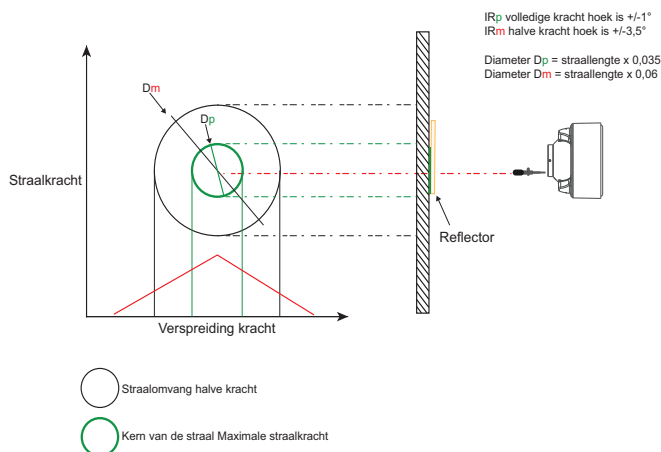
Afbeelding 2-18: Verdeling straalkracht
