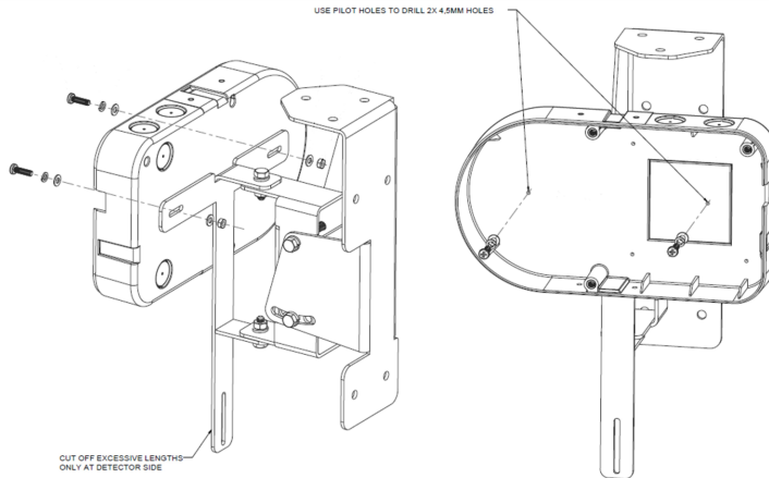
Figura 3-7: Linee guida per il montaggio del rivelatore
