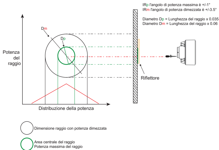
Figura 3-13: Distribuzione potenza raggio
