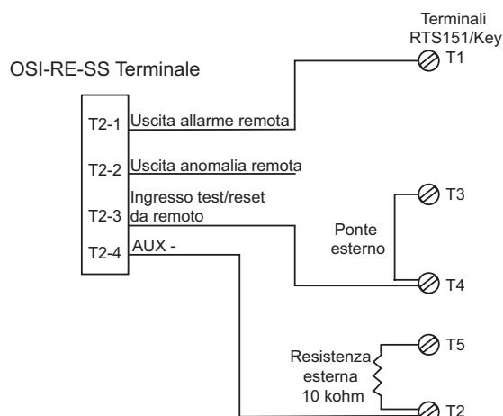
Figura 3-10: Schema elettrico (RTS451 o RTS151)
