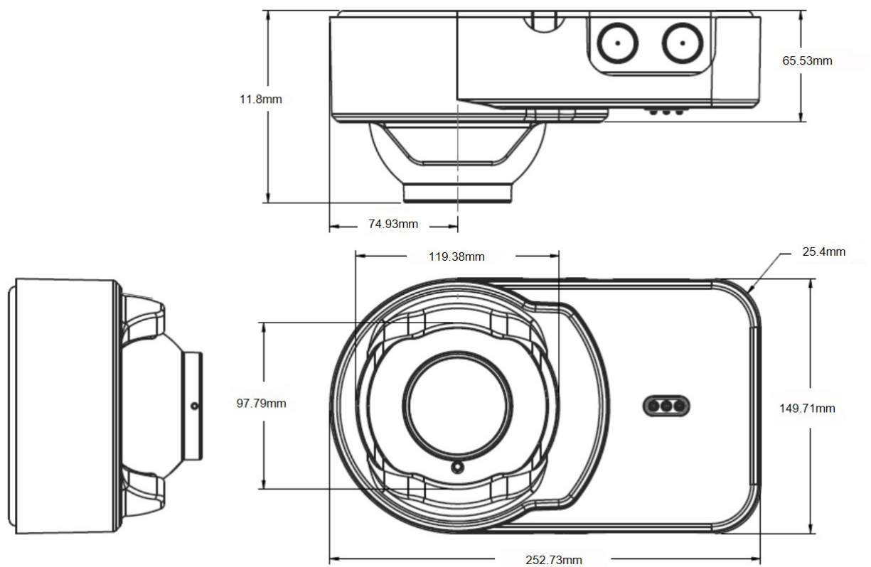
Figura 3-1: Dimensioni rivelatore
