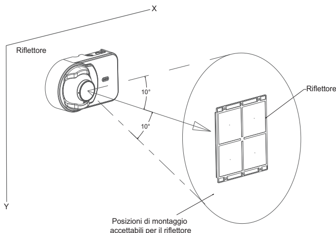
Figura 3-3: Linee guida per il montaggio del riflettore
