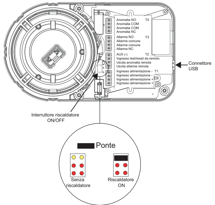
Figura 3-9: Connessioni elettriche presso il rivelatore
