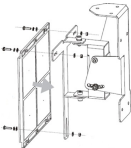
Figura 3-4: Linee guida per il montaggio del riflettore
