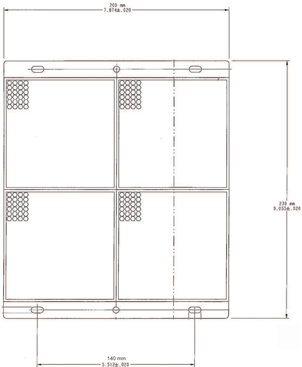
Figura 3-2: Dimensioni riflettore
