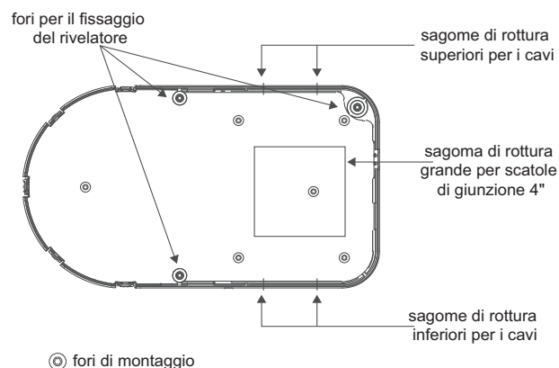
Figura 3-6: Fori di guida per il montaggio
