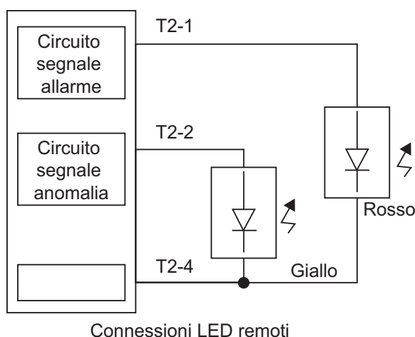
Figura 3-11: Schema elettrico (LED remoti)
