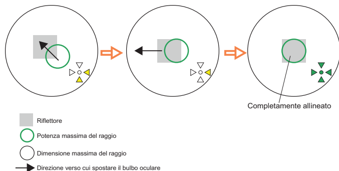
Figura 3-15: Guida a colori del set frecce per l'allineamento
