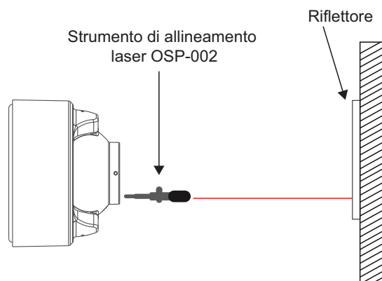
Figura 3-12: Allineamento grezzo
