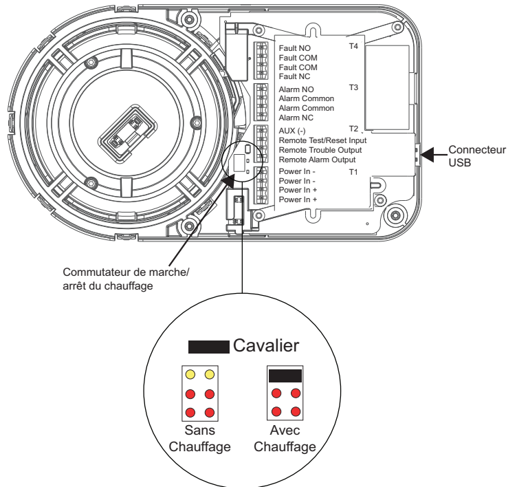
Figure 3-14: Raccords de câblage au détecteur
