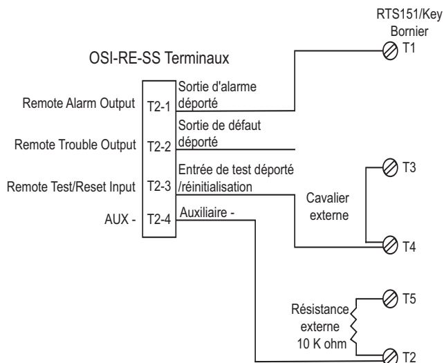
Figure 3-15: Schéma de câblage (RTS451 ou RTS151)
