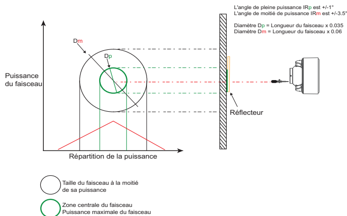
Figure 3-18: Répartition de la puissance du faisceau
