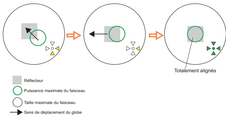
Figure 3-20: Guide d'alignement avec couleur de l'ensemble des flèches
