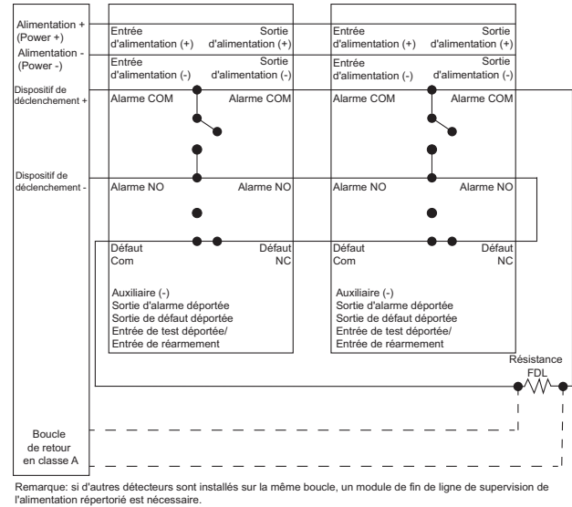
Figure 3-13: Schéma de câblage
