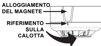
Figura 2: Montaggio del sensore sulla base
