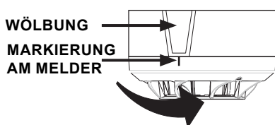
Abbildung 3a: Aktivierung der Entnahmesicherung
