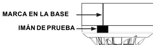
Figura 5: Posición del imán de prueba
