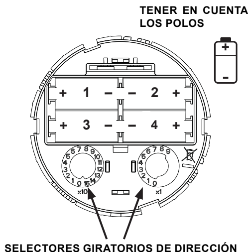
Figura 4: Instalación de las pilas y Selectores giratorios de dirección
