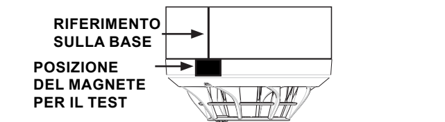
Figura 5: Posizione del magnete per il test
