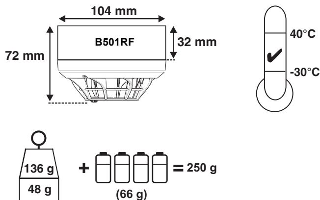
Abbildung 1: B501RF Montage
