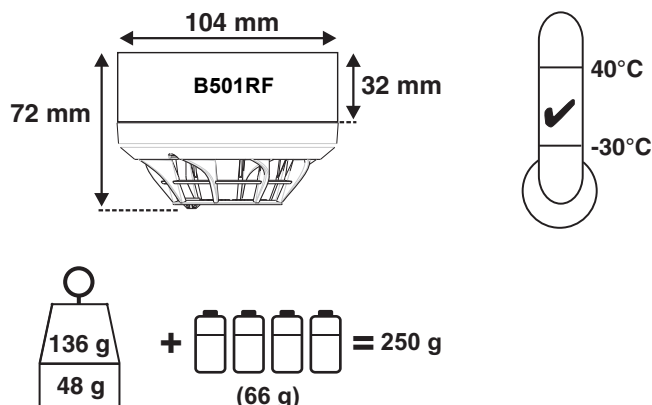
Figura 1: Montaggio B501RF
