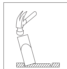
Figure 4: Comment perforez les orifices pour presse- étoupe
