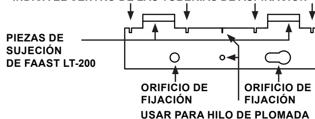
Figura 5: Soporte de montaje
