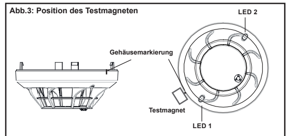
Abb.3: Position des Testmagneten
