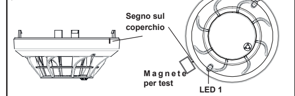
Figura 3: Posizione del magnete per il test
