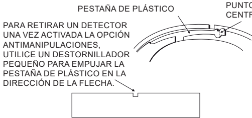
Figura 2: Opción de seguridad antimanipulaciones
