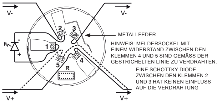
Abbildung 2: Sabotageschutz / Entnahmesicherung
