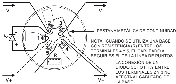
Figura 2: Opción de seguridad antimanipulaciones
