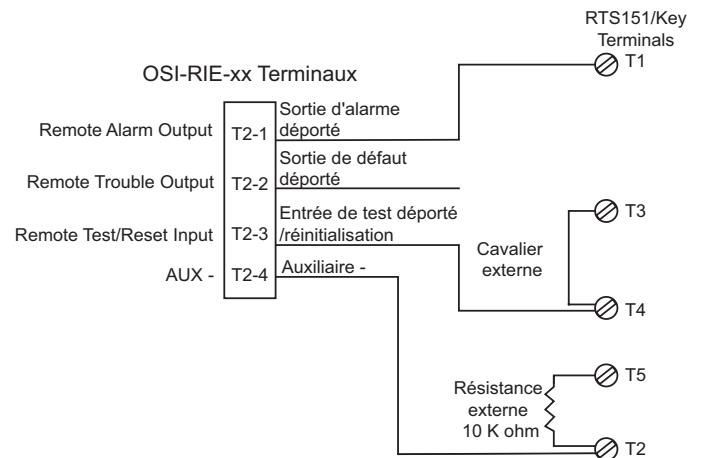
Figure 4-15: Schéma de câblage (RTS151)
