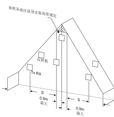
图 1-6: 倾斜天花板(尖顶型)
