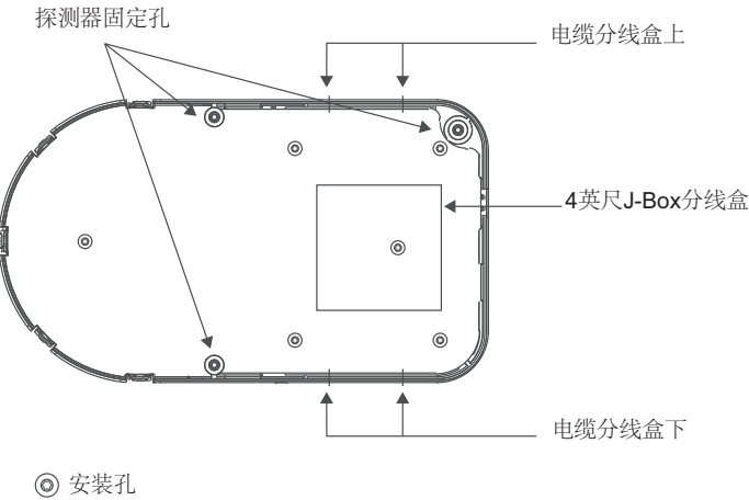
图 1-11: 安装导孔
