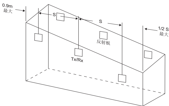
图 1-5: 倾斜天花板(棚屋型)
