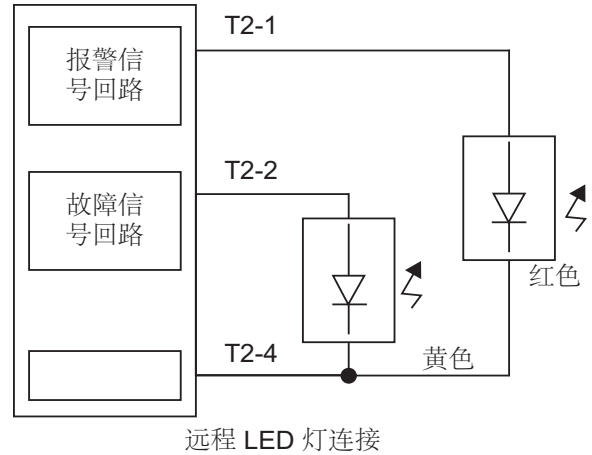
图 1-16: 接线示意图(远程 LED 灯)
