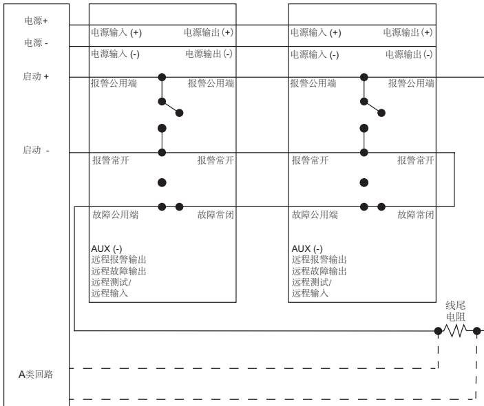
图 1-13: 接线示意图
