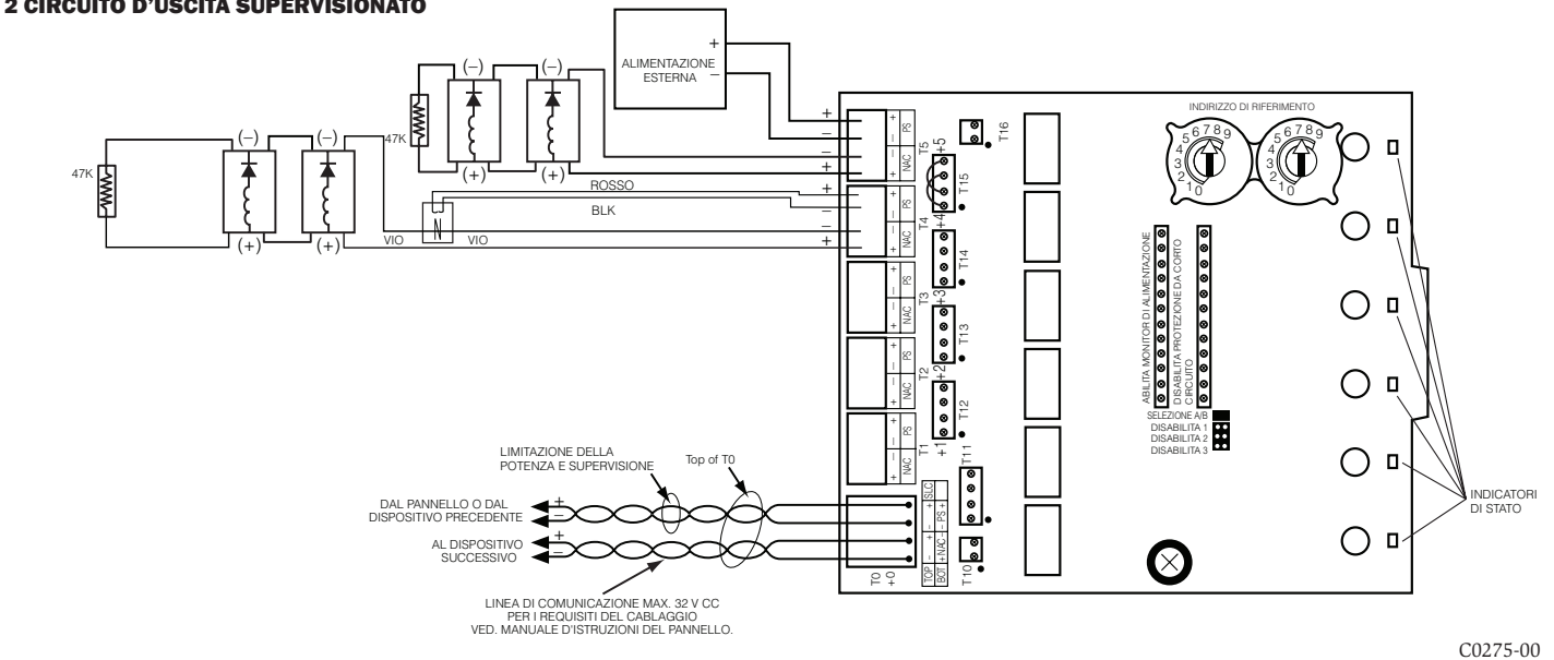
FIGURA 3. ESEMPIO DI CONFIGURAZIONE CIRCUITO D'USCITA SUPERVISIONATO CLASSE B CON UN SINGOLO ALIMENTATORE CONDIVISO DA 2 CIRCUITO D'USCITA SUPERVISIONATO
