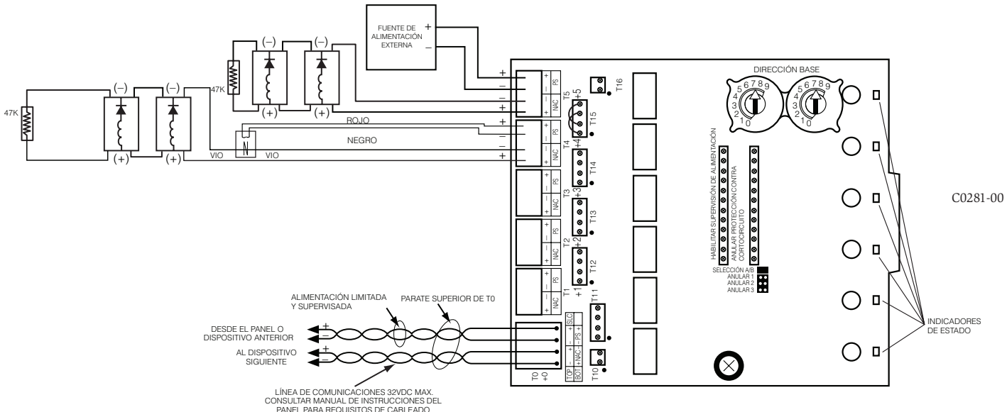
FIGURA 3. EJEMPLO DE CONFIGURACIÓN DEL CIRCUITO DE SALIDA SUPERVISADO EN CLASE B CON UNA ÚNICA FUENTE DE ALIMENTACIÓN COMPARTIDA POR DOS CIRCUITOS DE SALIDA SUPERVISADOS
