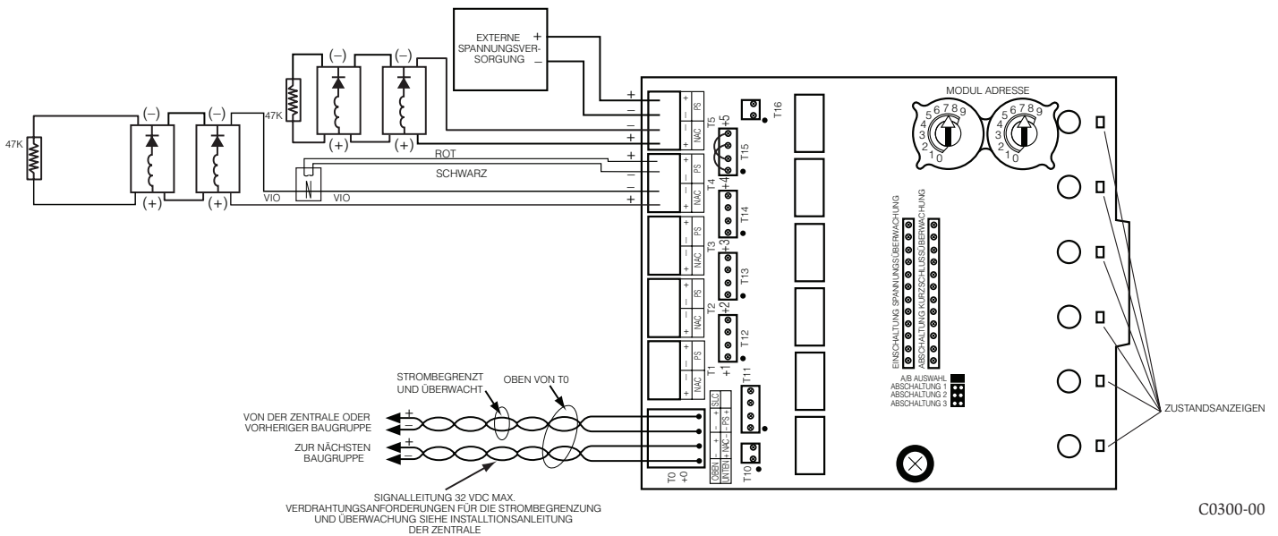
ABBILDUNG 3. KONFIGURATION DER ÜBERWACHTEN STEUERAUSGÄNGE MIT EINER EINZIGEN SPANNUNGSVERSORGUNG FÜR 2 ÜBERWACHTETE STEUERAUSGÄNGE
