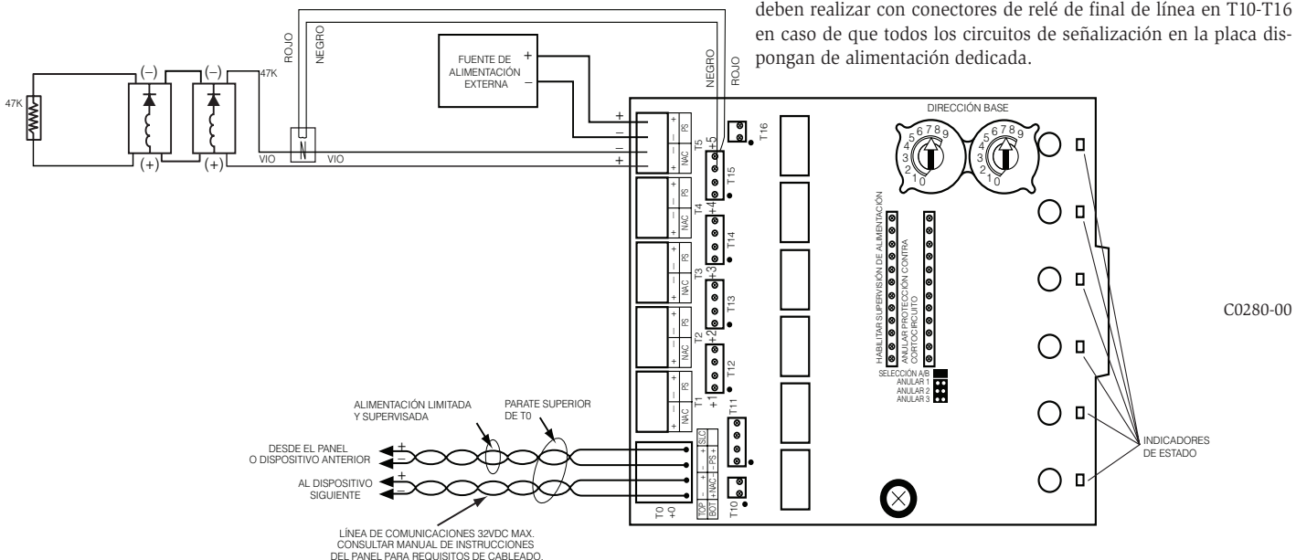
FIGURA 3. EJEMPLO DE CONFIGURACIÓN DEL CIRCUITO DE SALIDA SUPERVISADO EN CLASE B CON UNA ÚNICA FUENTE DE ALIMENTACIÓN COMPARTIDA POR DOS CIRCUITOS DE SALIDA SUPERVISADOS
