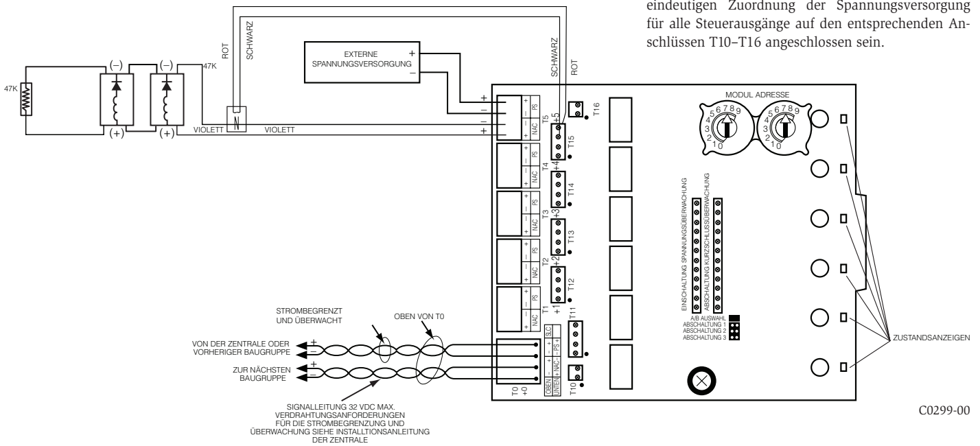
ABBILDUNG 3. KONFIGURATION DER ÜBERWACHTEN STEUERAUSGÄNGE MIT EINER EINZIGEN SPANNUNGSVERSORGUNG FÜR 2 ÜBERWACHTETE STEUERAUSGÄNGE
